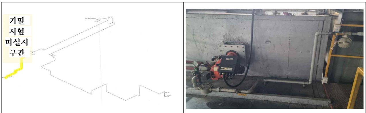
[ 그림 3 ] ‘H’ 2차조정기 출구측 배관 기밀시험 미실시 구간 현황
